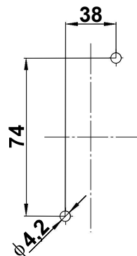
Stražnji lim (samo za izvedbu "O") Rear plane (only for option "O")
